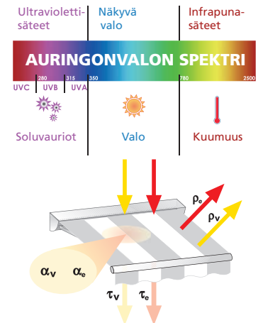
Kuva näyttää symbolit: läpäisy r (Tau), heijastus p (Rho), valon spektrin laskennallisen arvon v , näkyvän valon e eristyksen ja näkyvän valon absorptiota a (alpha). Punainen nuoli kertoo lämpösäteilystä ja keltainen nuoli näkyvästä valosta
